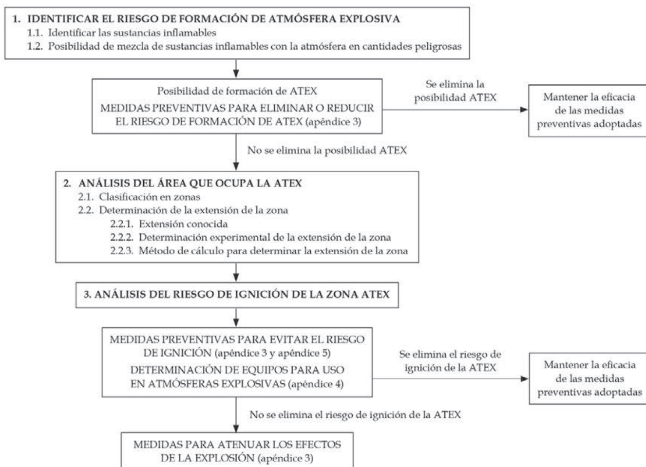
Figura 7. Diagrama del conjunto de actividades preventivas que se deben realizar en zonas con riesgo de ATEX.
